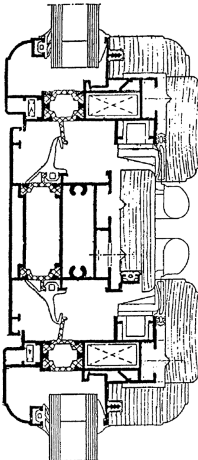
Рисунок 12 - Примеры конструктивного решения профильных систем
